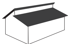
PULTDACH ERWEITERT/VERSETZT
